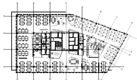
Piętro 1 | Floor 1
